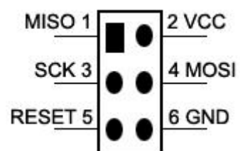
6-pin ISP 介面定義
